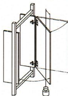
Схема испытания на долговечность
